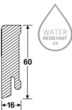
Fußleiste Profil 23 F MK
